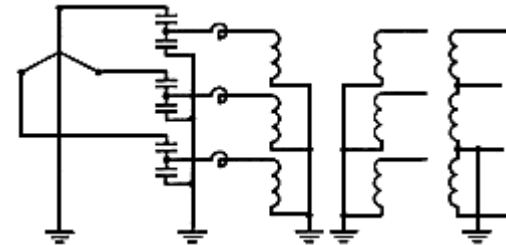
Рисунок Б.10 - Схема включения однофазных емкостных трансформаторов напряжения в трехфазных электрических сетях с заземленной нейтралью и напряжением 110 кВ и выше
