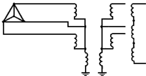
Рисунок Б.3 - Схема включения однофазных заземляемых и трехфазных заземляемых двухобмоточных трансформаторов в трехфазных электрических сетях с изолированной нейтралью и напряжением 3-35 кВ
