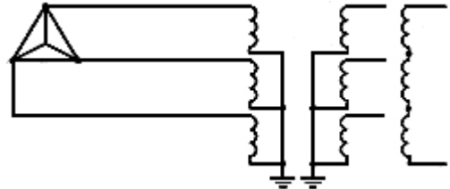
Рисунок Б.2 - Схема включения однофазных заземляемых и трехфазных заземляемых двухобмоточных трансформаторов в трехфазных электрических сетях с изолированной нейтралью и напряжением 3-35 кВ
